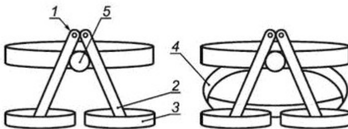
Рисунок 1 - Примеры компоновок элементов привязи для положения сидя
