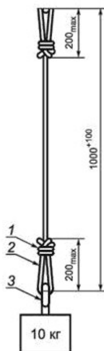
Рисунок 3 - Строп для определения динамических характеристик
