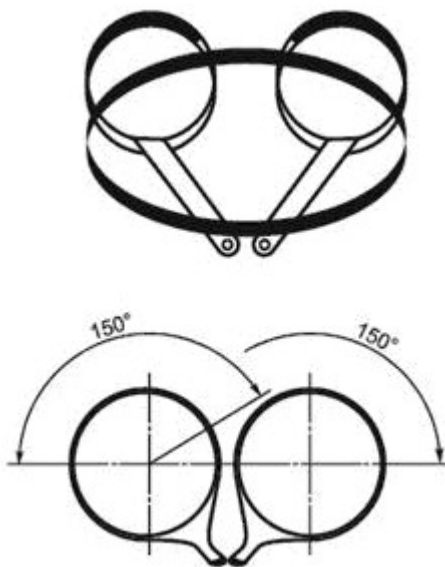
Части ремней, несущие нагрузку
